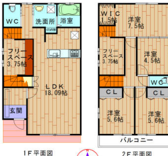
1F平面図
